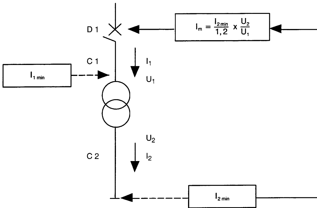
Figure 1 – Protection de la canalisation C 2 assurée par le dispositif D 1 (à condition que I_m \leq I_1 \text{ minimal} )
